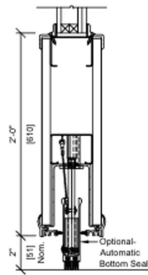
Optional Automatic Bottom Seal
